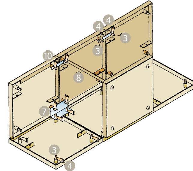
FIGURA 2 Pareti Lineari
